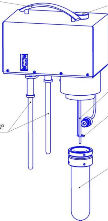
Рисунок 3 – Блок технологический
