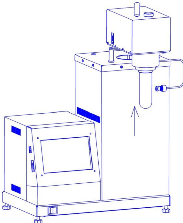
Рисунок 9 – Установка колбы
