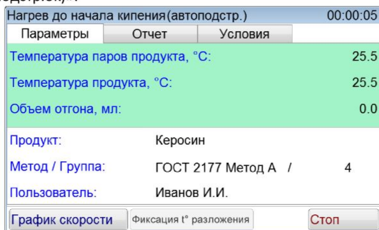
Рисунок 71 – Испытание с автоподстройкой
