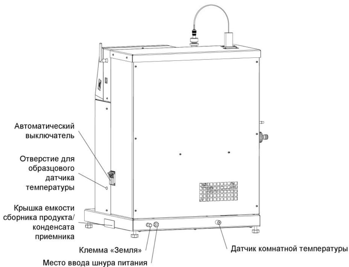
Рисунок 3 – Вид аппарата сзади
