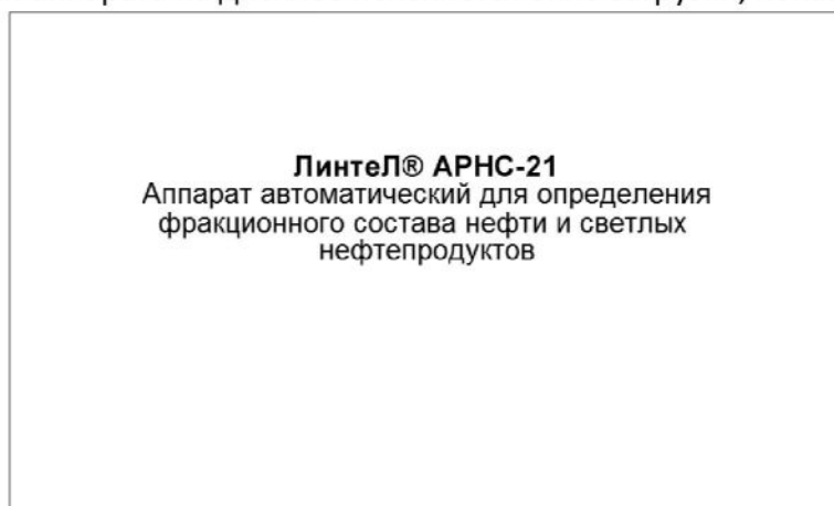
Рисунок 5 – Окно загрузки
