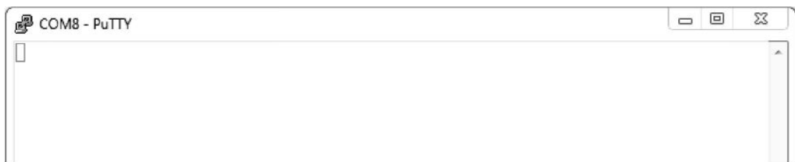
Рисунок 84 – Окно терминала
