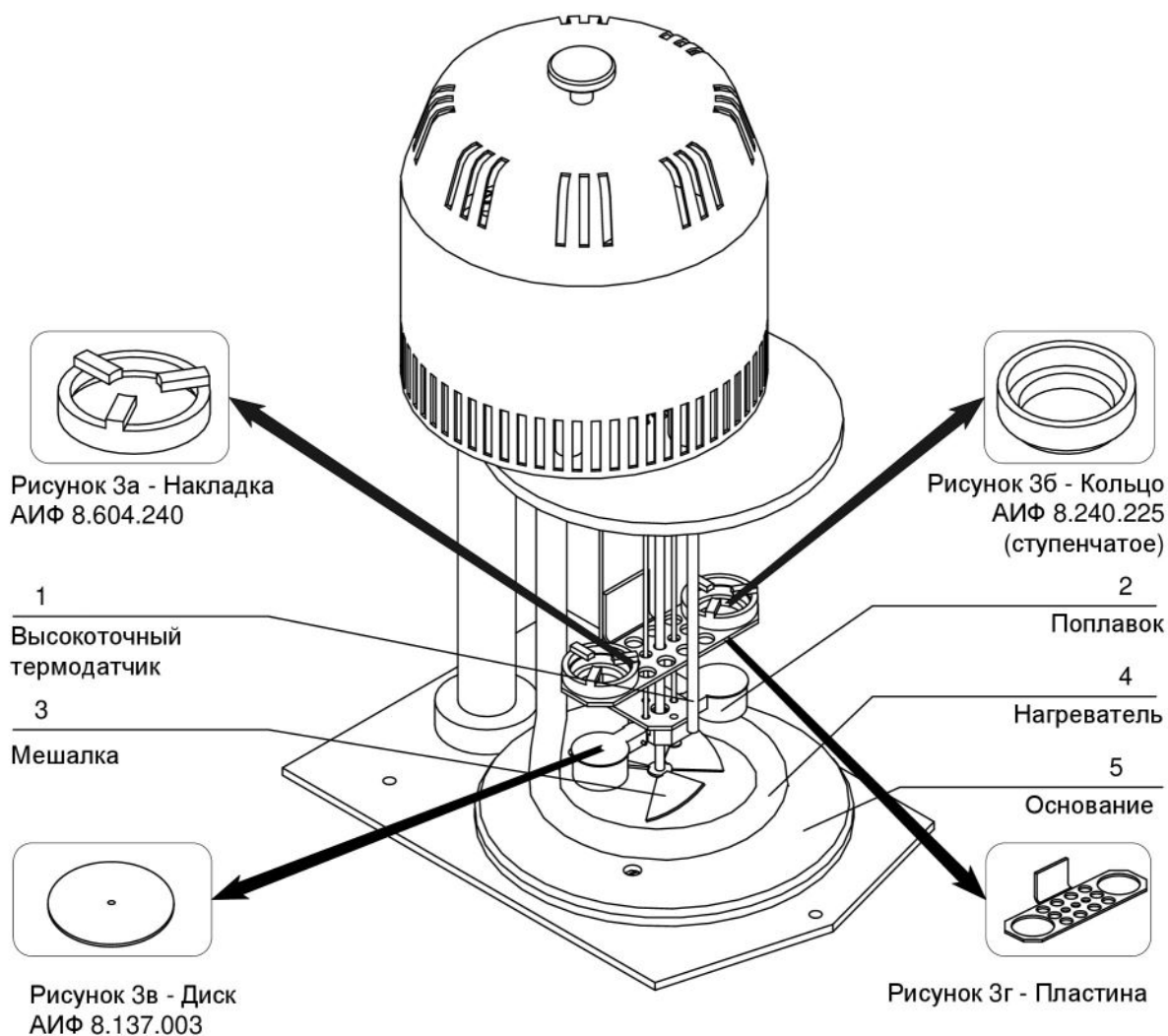
Рисунок 3 – Технологический блок
