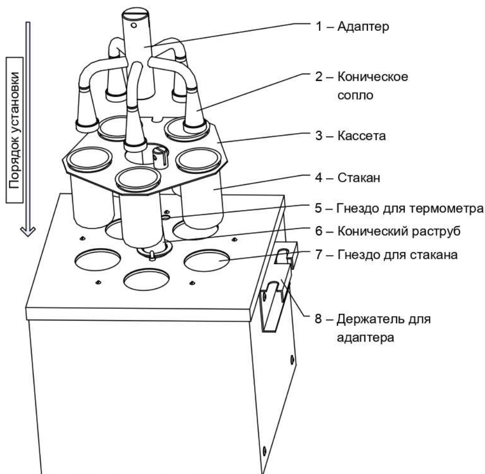
Рисунок 3 – Технологический блок
