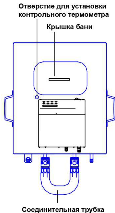
Рисунок 3. Вид сверху
