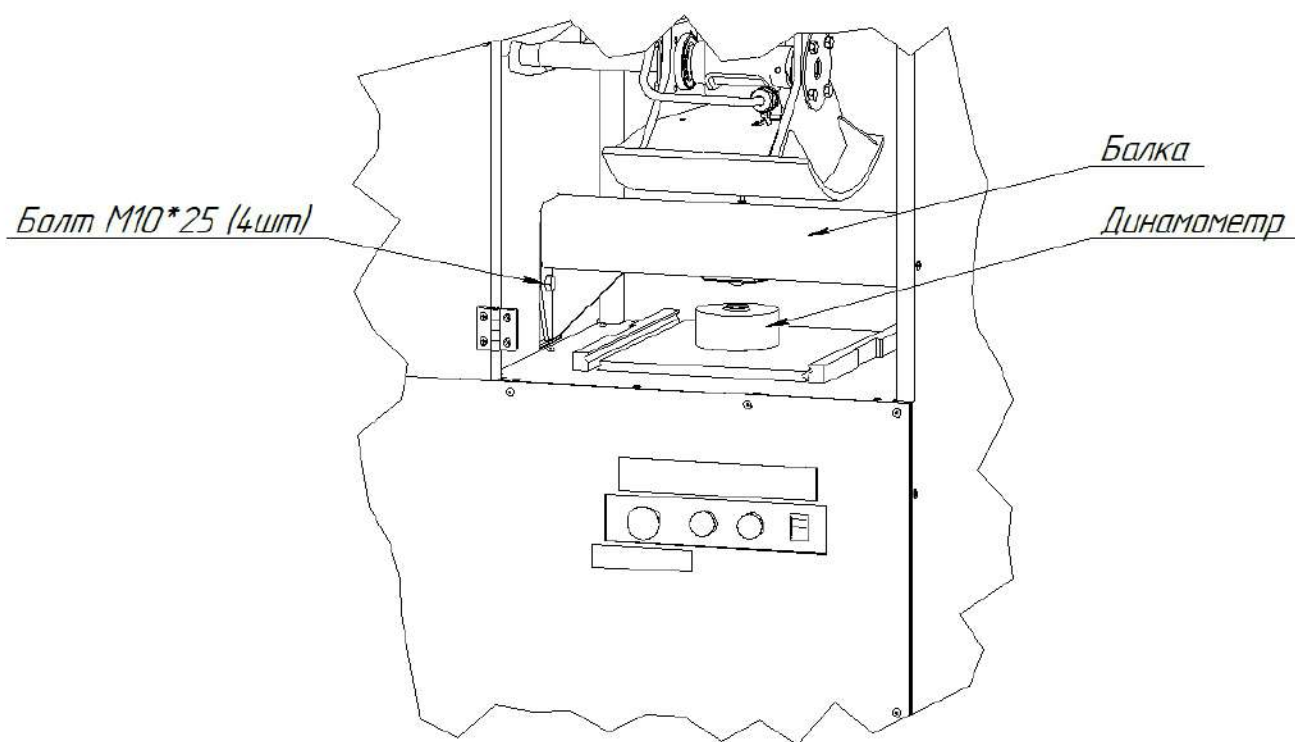
Рисунок 13 – Установка балки
