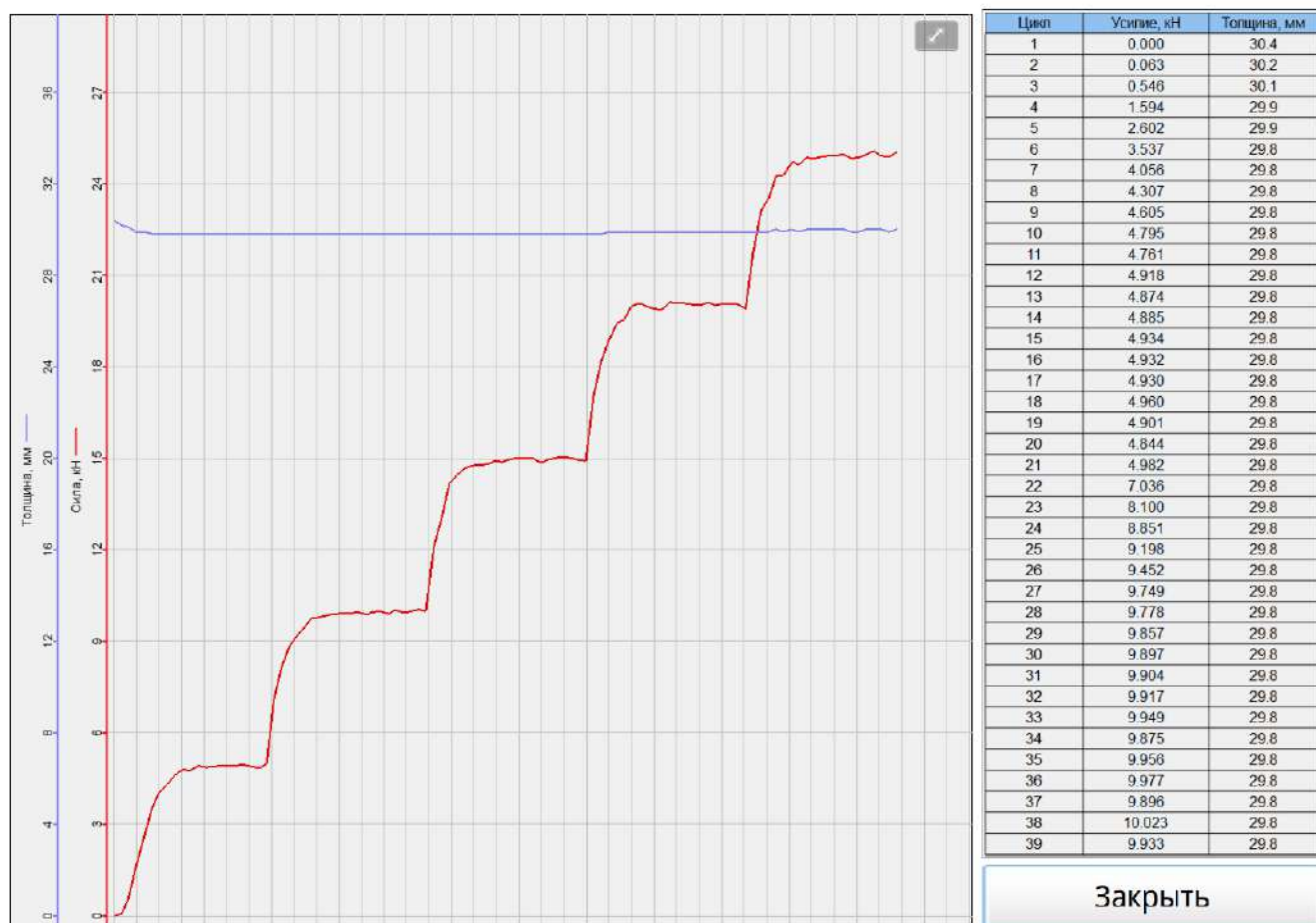
Рисунок 10 – Просмотр графиков
