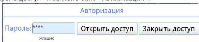
Рисунок 14 – Окно авторизации
