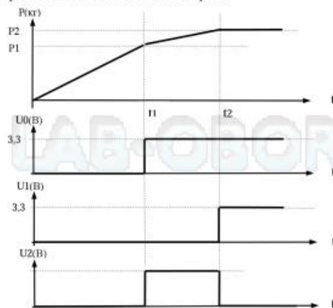
Табл. 4.2 - Диаграмма сигналов управления заслонками дозатора
