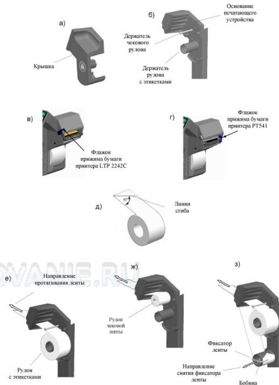
Рис. 2.3 - Установка рулонов в терминалах RP и R2P
