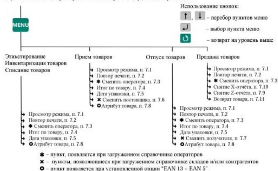
Рис. 7.1 - Структура меню оператора
