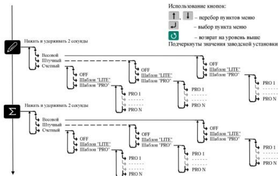
Рис. 4.2 - Схема установки шаблонов печати
