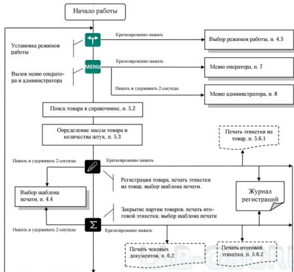
Рис. 3.1 - Схема работы терминала RP (R2P)
