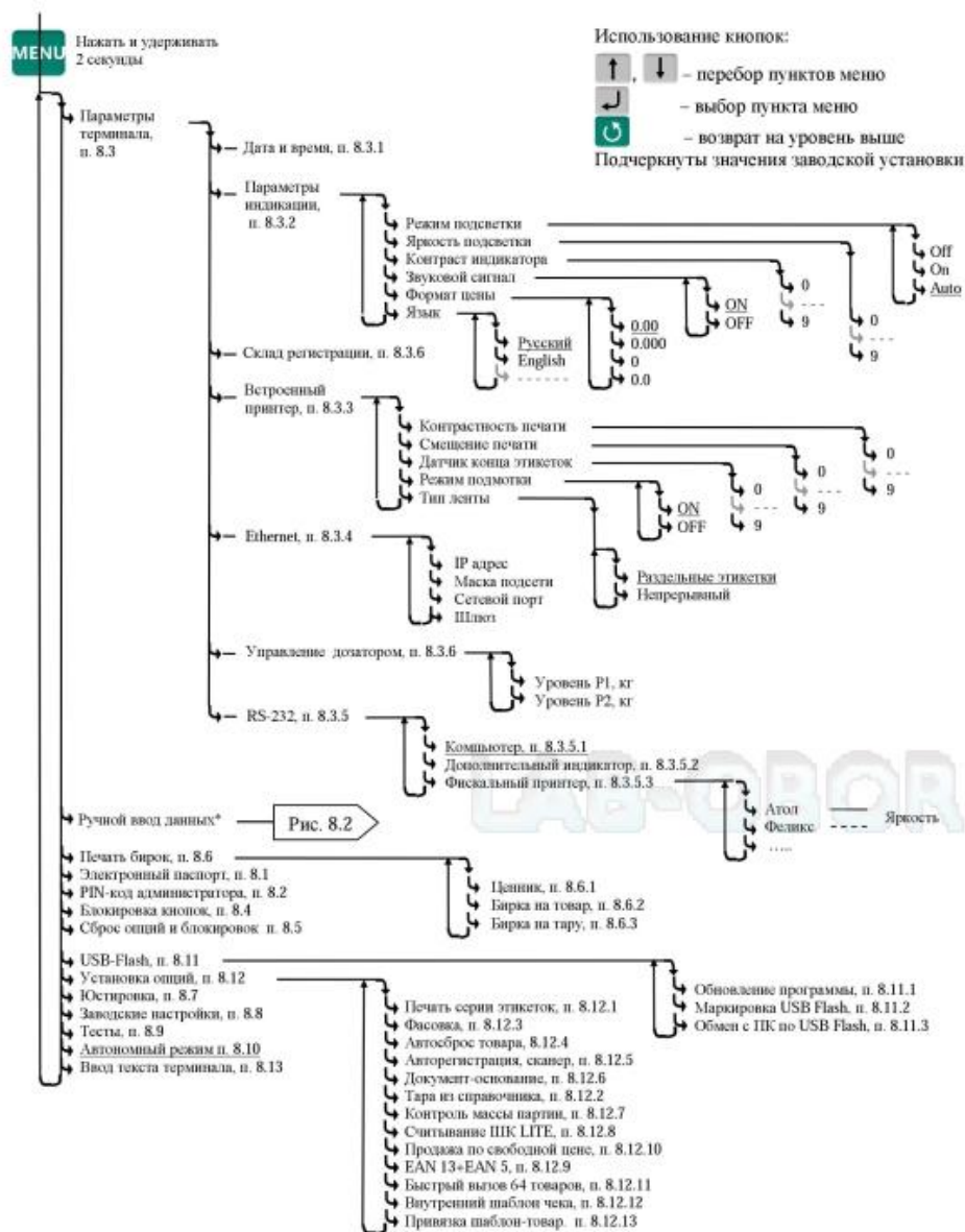
Рис. 8.1 - Структура меню администратора
