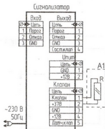
R – имитатор клапана (резистор типа C2-33-0, 125-100 Ом-20%) Рисунок В.1 – Одиночный сигнализатор
