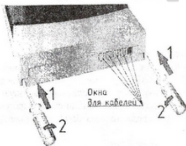
Рисунок 2 – Снятие крышки клеммного отсека
