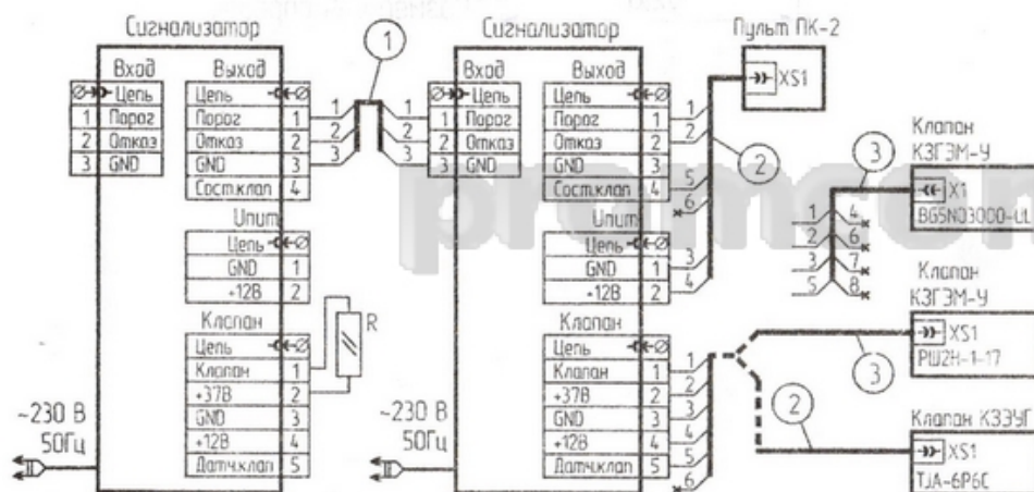
R – имитатор клапана (резистор типа C2-33-0, 125-100 Ом-20%) 1 – Кабель типа КСПВ 4х0,52 (UTP-2) 2 – Кабель ЯБКЮ.685611.108-02 3 – Кабель ЯБКЮ.685611.009 (ЯБКЮ.685611.109)
