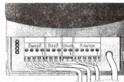
Рисунок 4 – Расположение разъемов
