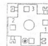
Розетка G2U3000-SK-1G нумерация контактов со стороны монтажа
