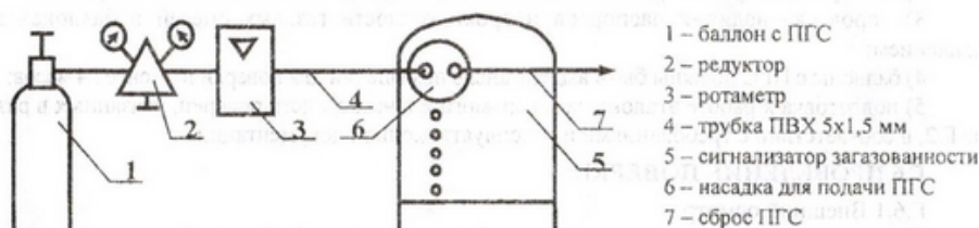
Рисунок Г.1 – Схема для настройки и проверки сигнализатора с применением ПГС
