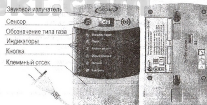
Рисунок 1 – Внешний вид сигнализатора
